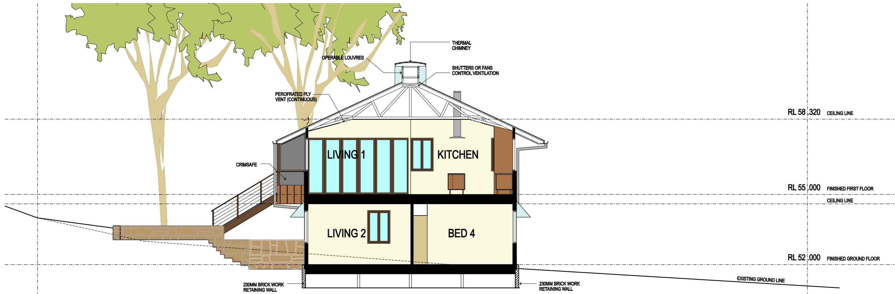
SECTION A-A
