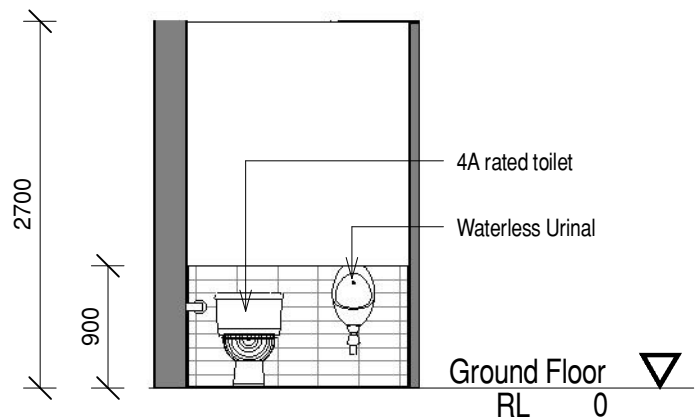
D PWD - Elevation D 1 : 50
